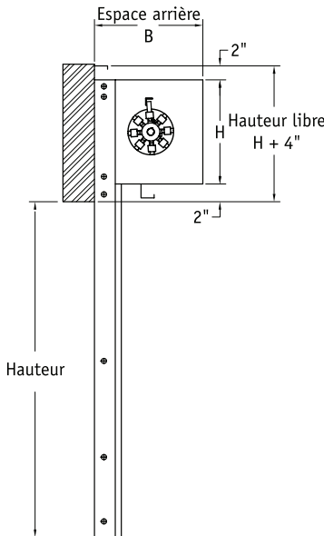
GRAPHIQUE À DEUX DIMENSIONS* Porte de service de la série 6000
