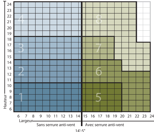
GRAPHIQUE À DEUX DIMENSIONS* Porte de service de la série 6000
