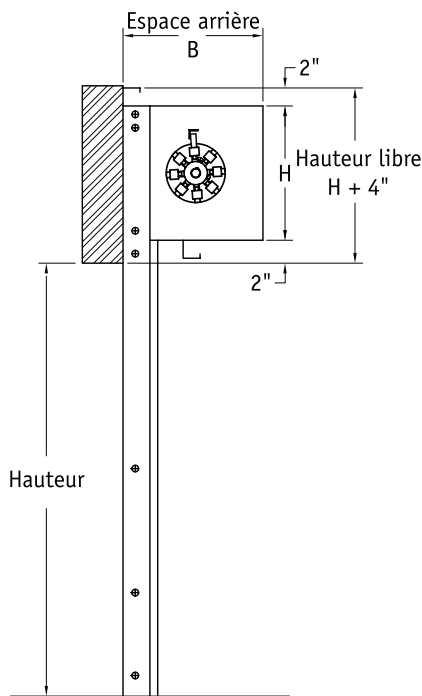
GRAPHIQUE À DEUX DIMENSIONS* Portes de service modèle 6241
