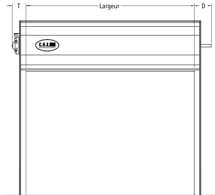
GRAPHIQUE À DEUX DIMENSIONS* Portes de service modèle 6241
